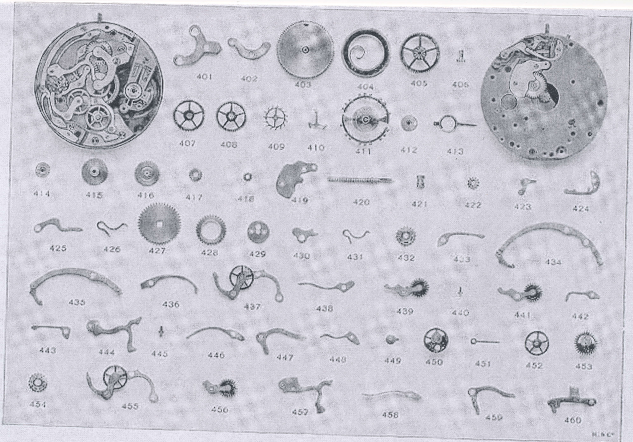
Pièces de rechange pour Chronographe Cal. 14 me G.H.
